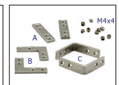
Connector(optional) A) Direct B) 90° inside C) 90° outside
